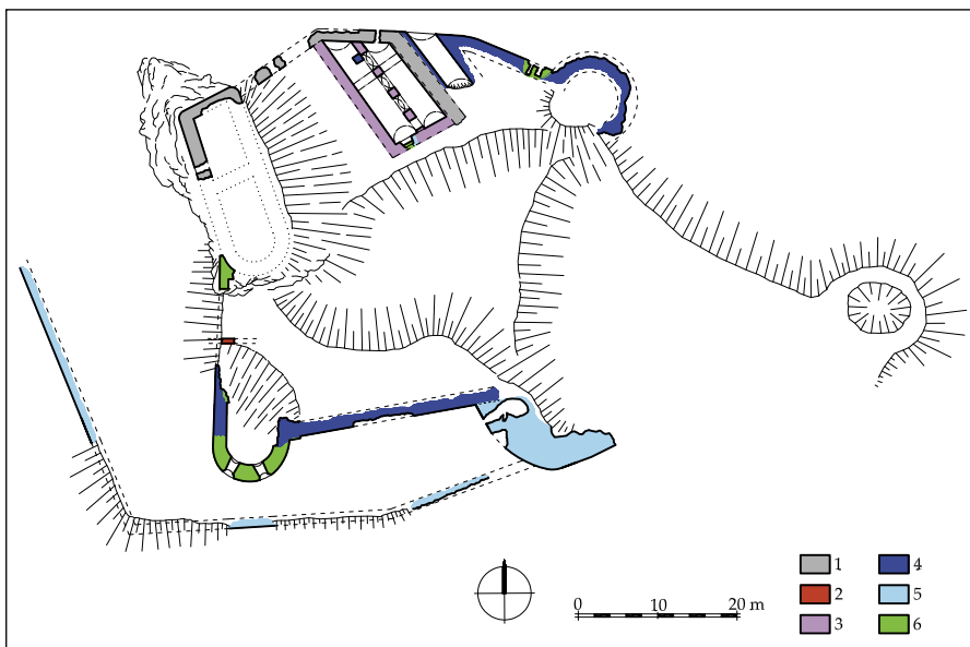
Obr. 140. Pôdorys hradu Plaveč s naznačením jednotlivých etáp výstavby: 1 – druhá polovica 13. až začiatok 14. storočia; 2, 3 – 14. a 15. storočie; 4, 5 – 16. storočie, 6 – 18. a 19. storočie.
