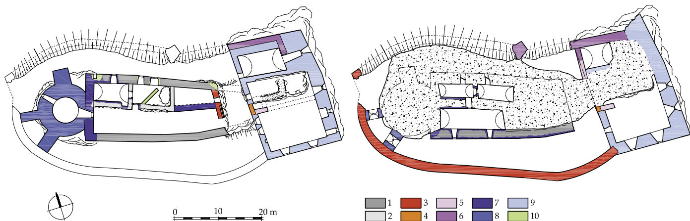
Obr. 143. Pôdorys jadra hradu Lubovňa v úrovni prízemnia s naznačením jednotlivých etáp výstavby: 1, 2 – 14. storočie; 3 – koniec 14. až prvá polovica 15. storočia; 4, 5, 6 – 15. storočie; 7 – koniec 15. až začiatok 16. storočia; 8 – prvá tretina 16. storočia; 9 – okolo polovice 16. storočia; 10 – mladšie.
