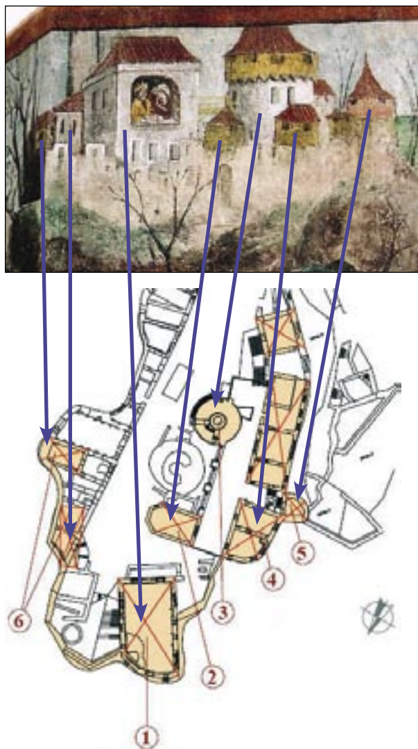
Obr. 148. Vyznačenie zástavby na vrchnom nádvorí Spišského hradu na začiatku 16. storočia: 1) románsky palác s oknom po gotickej prestavbe, 2) kaplnka, 3) kruhová veža po gotickej úprave a nadstavbe, 4) Paláce Zápoľskovcov – Dom kaplánov, 5) Okrúhla „Červená veža“, 6) Objekty – Východné krídlo.
