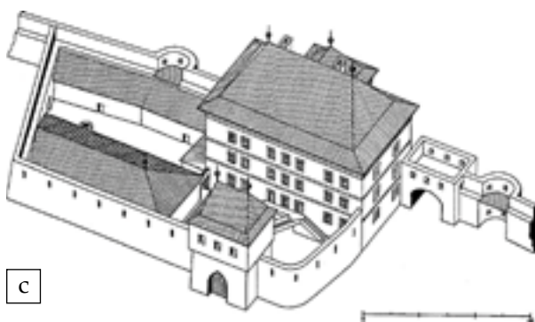
Obr. 151. a) Pôdorys Podolínca s vyznačeným mestským hradom, b) pôdorys hradu, c) ideálna rekonštrukcia hradu v 18. storočí.
