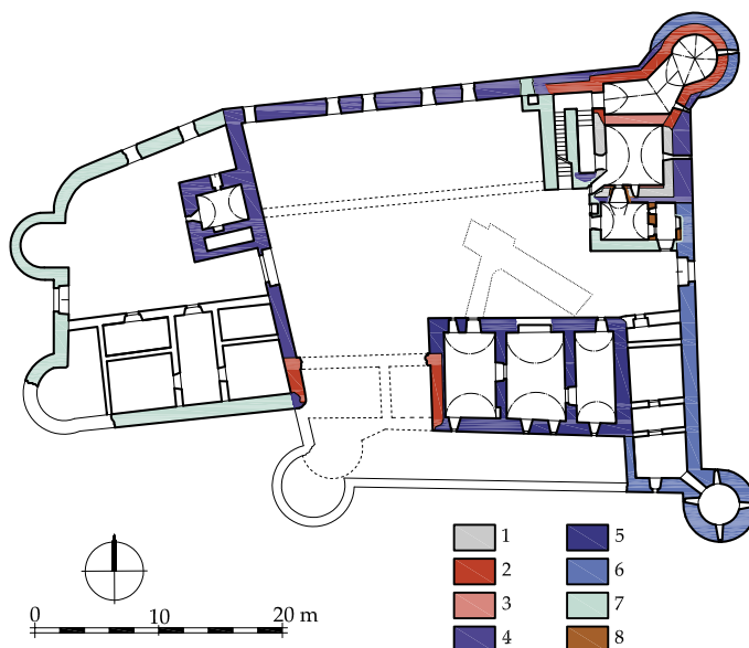
Obr. 165. Markušovce. Celkový pôdorys s rozkreslením jednotlivých fáz. 1 – 14. – 15. storočie, 2 – začiatok 16. storočia, 3 – pred rokom 1569, 4 – 7 – druhá polovica 16. storočia až 17. storočie, 8 a biele – mladšie.
