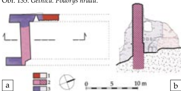
Obr. 136. Gelnický hrad, a) pôdorys a b) rez paláцovej budovy na južnej strane.
